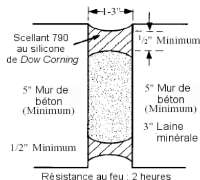
Schéma 1 : Construction d'un joint extérieur et résistance au feu (selon la norme UL 263, ASTM E 119)
