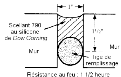
Schéma 1 : Construction d'un joint extérieur et résistance au feu (selon la norme UL 263, ASTM E 119)
